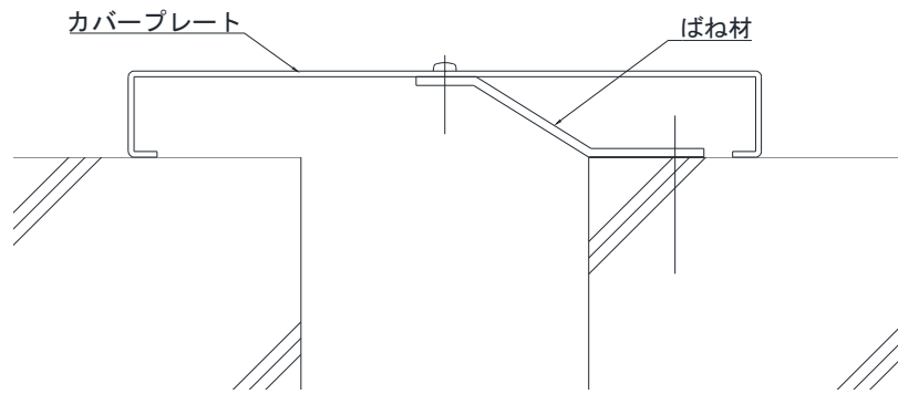
躯体間クリアランスの納まり概念図
