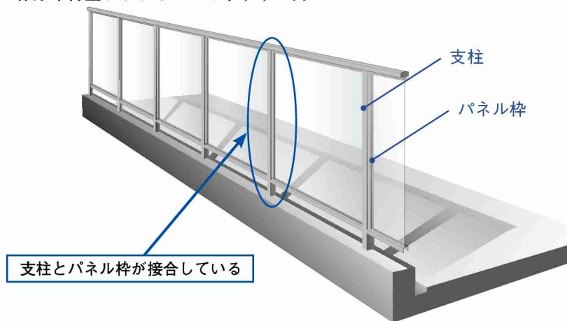
図7 支柱に一樣分布荷重がかかるアルミ手すりの例
