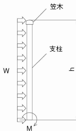
図9 風荷重イメージ
