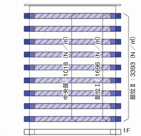
図4 建築物各階層の設計風圧力
