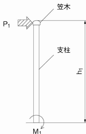
図8 支柱頂部への集中荷重イメージ
