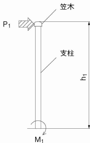
図11 支柱頂部への集中荷重イメージ
