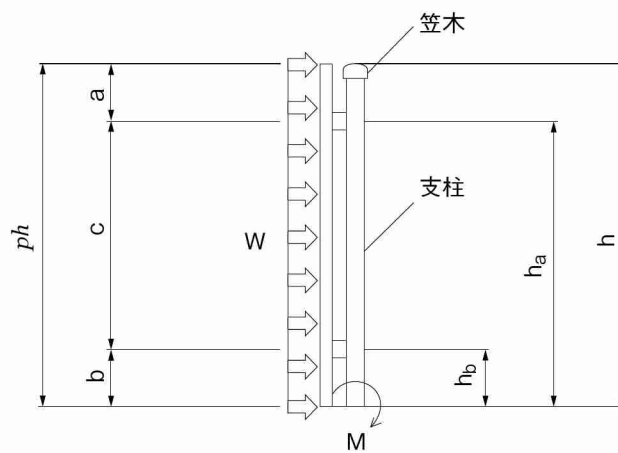
図12 風荷重イメージ
